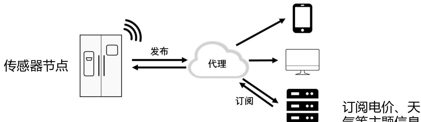
MQTT协议示意图
