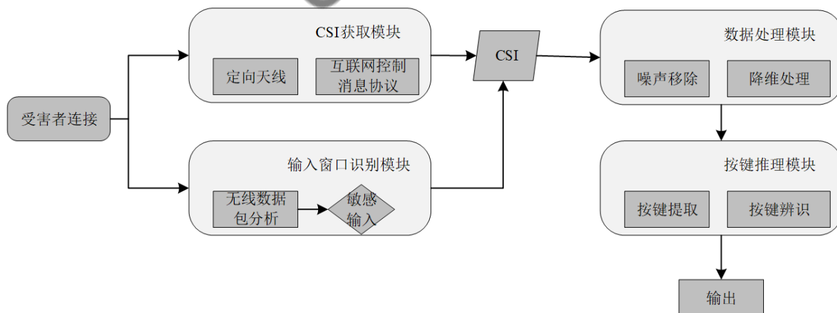
WindTalker框架图示
